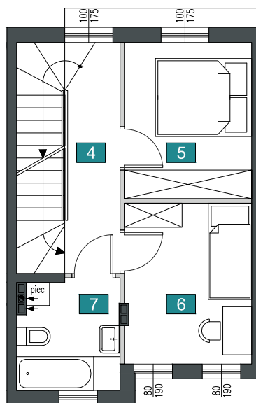
RZUT PIĘTRA
